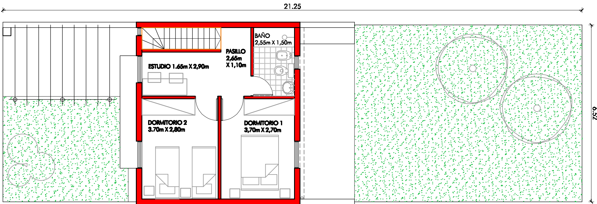
Planta Alta 2 Dormitorios + Estudio 40m 2
